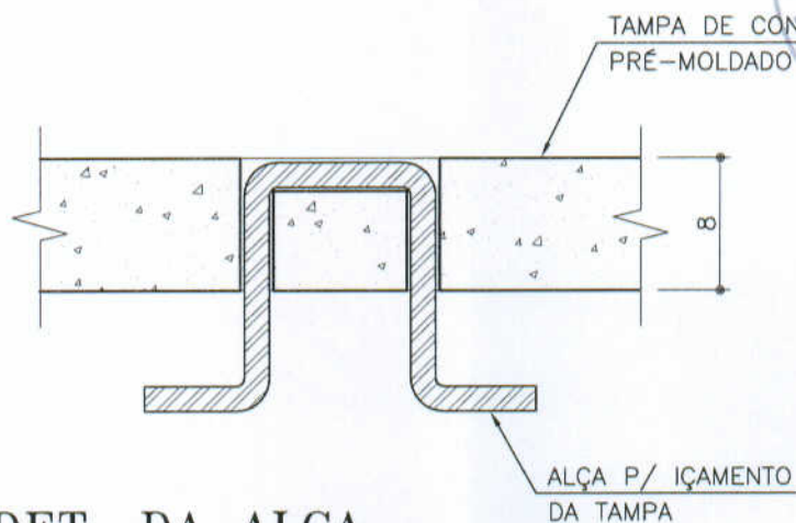
4 DET. DA ALÇA ESCALA 1:5
