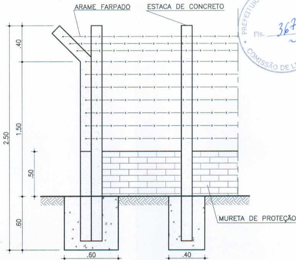
CORTE-AA Escala: 1/25
